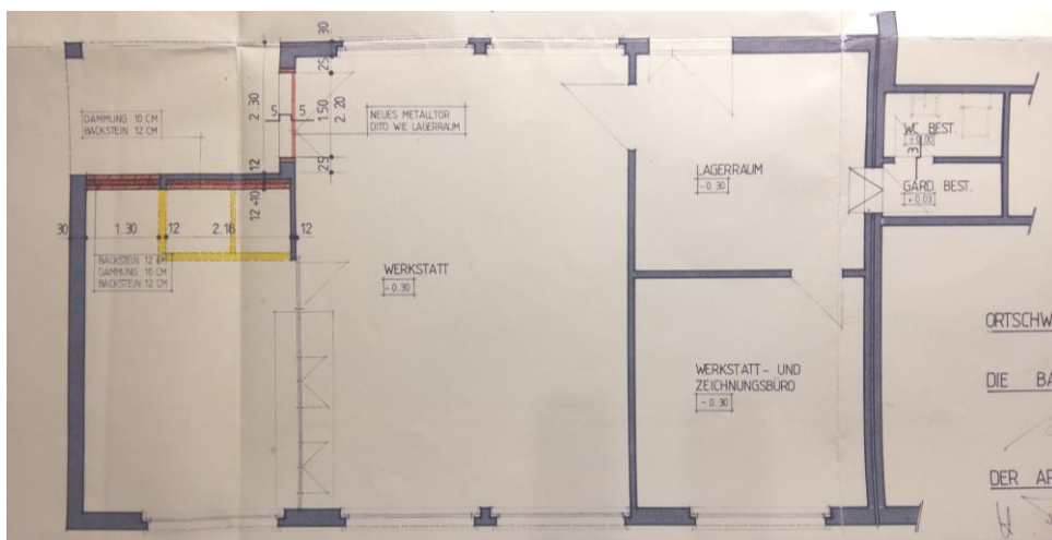
Grundriss
